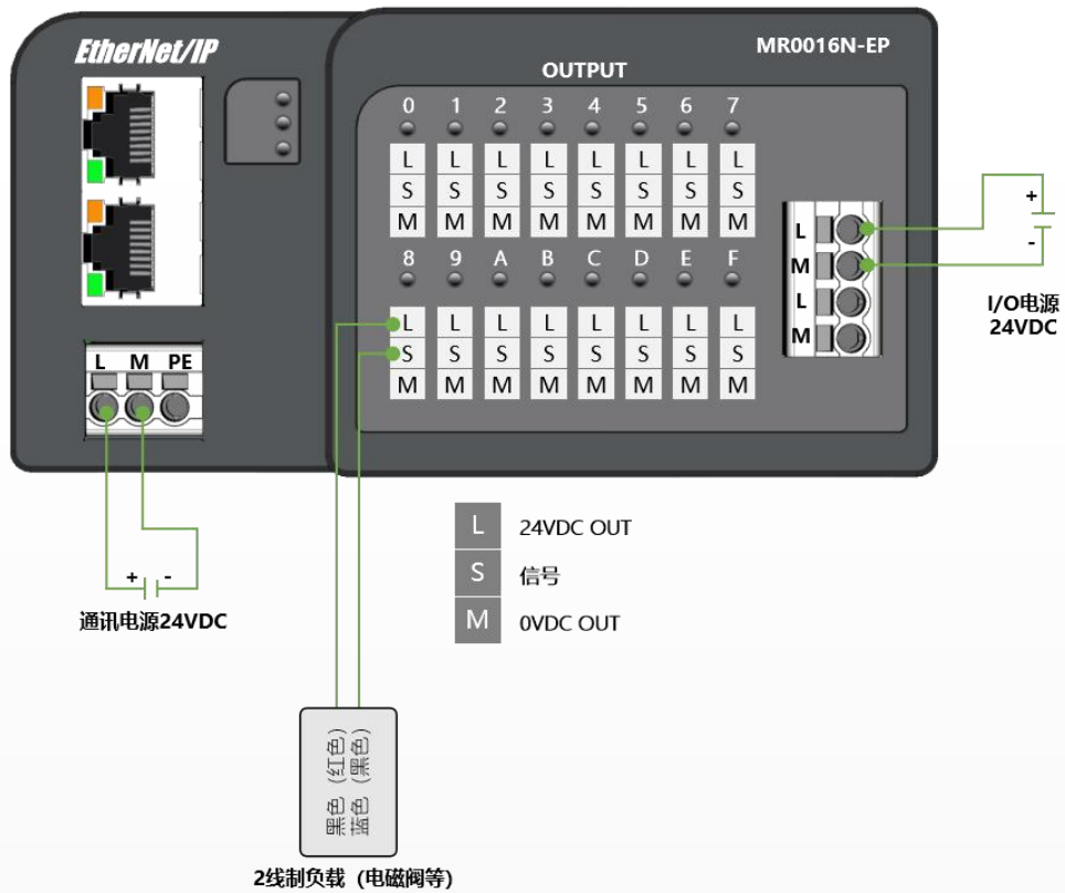
16 点输出 NPN
