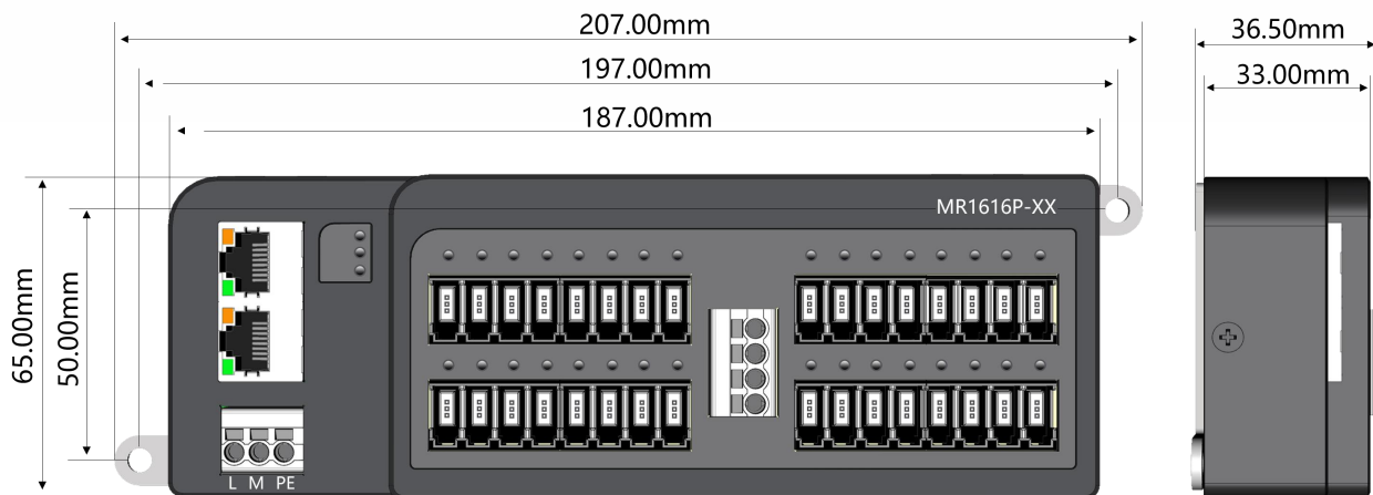
图 4 尺寸 1--207 *65 (W/H, mm)
