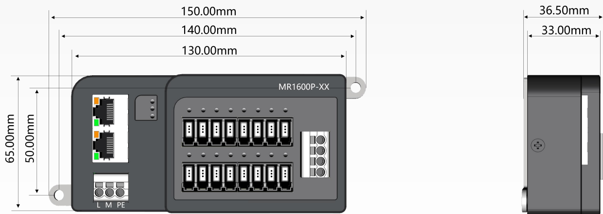
图 3 尺寸 150 *65 (W/H, mm)
