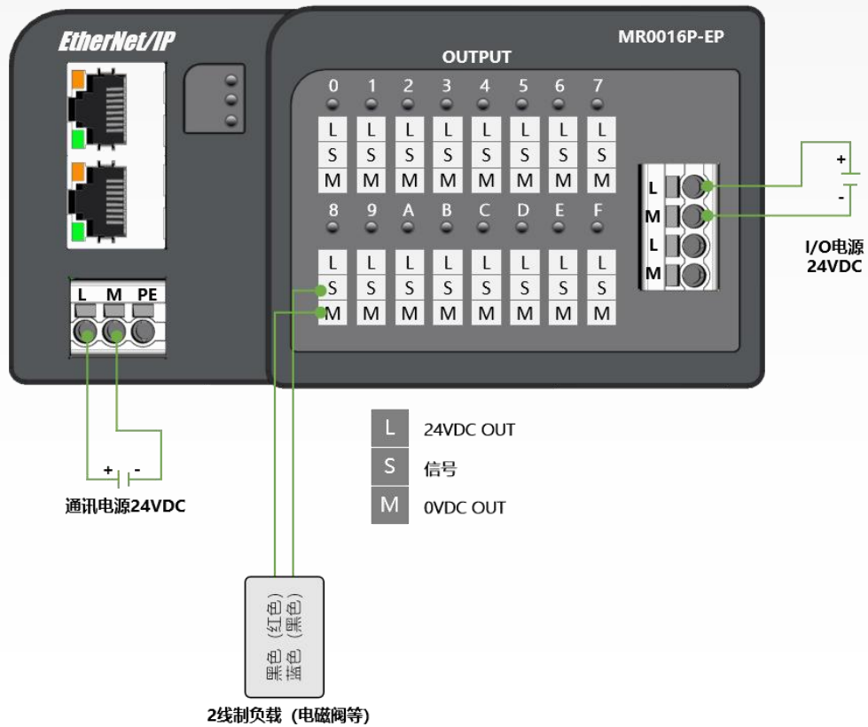
16 点输出 PNP
